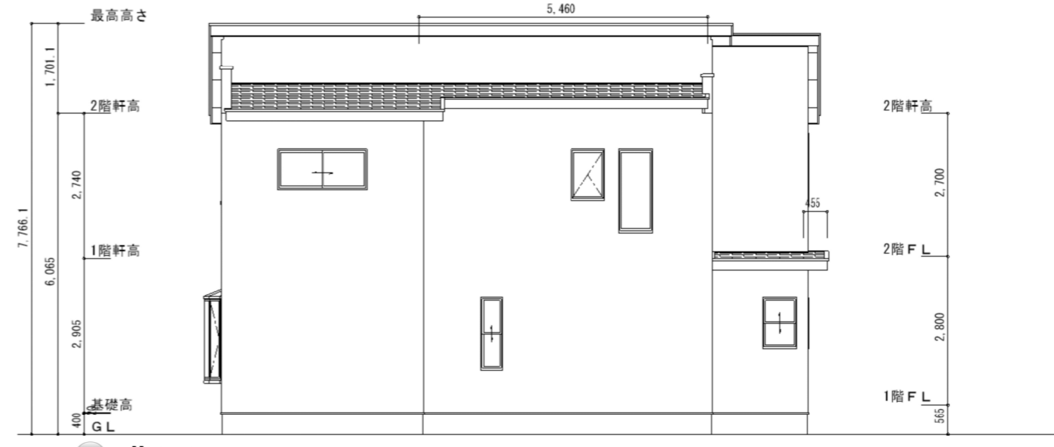
● 北面
