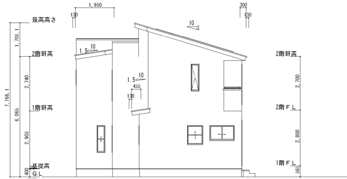
● 西面
