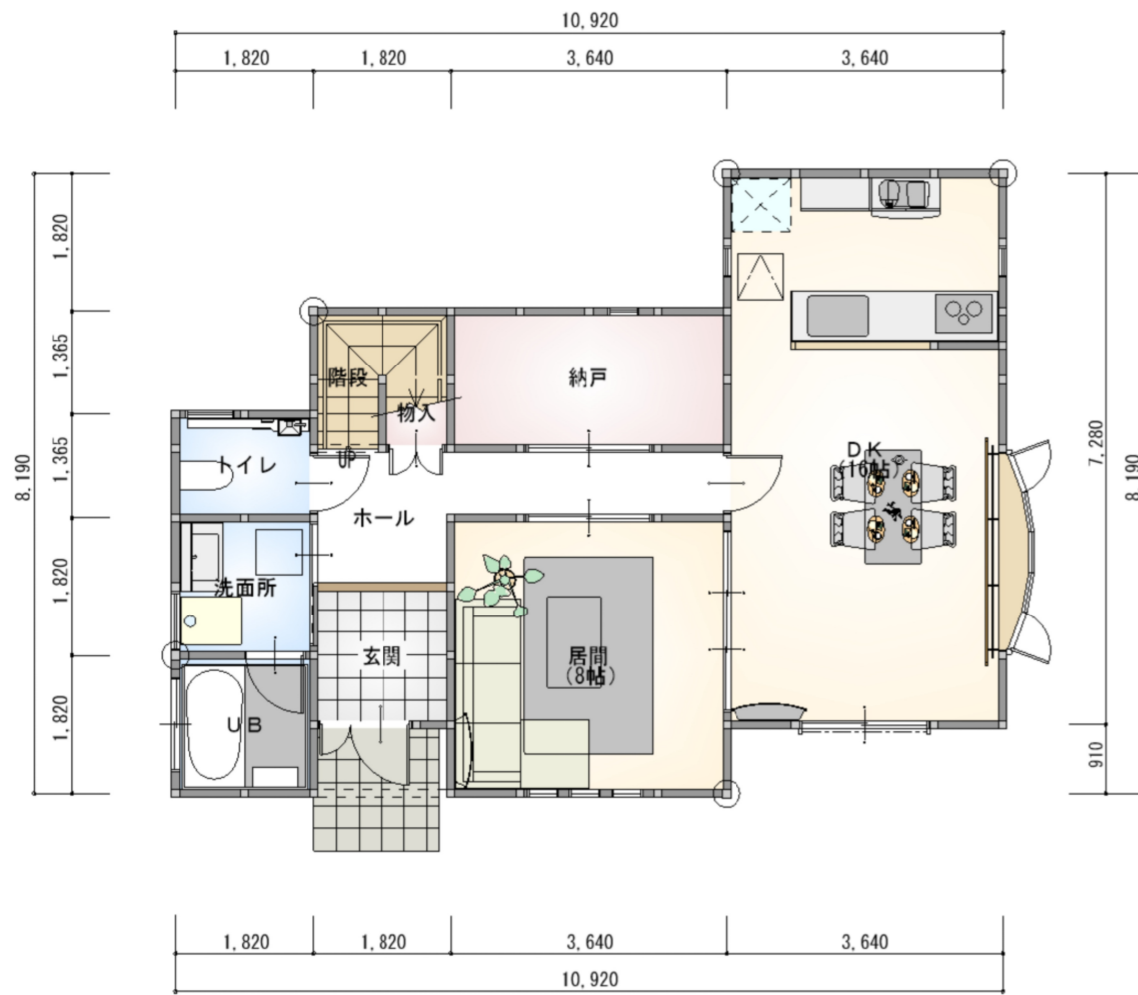
● 1階平面図
