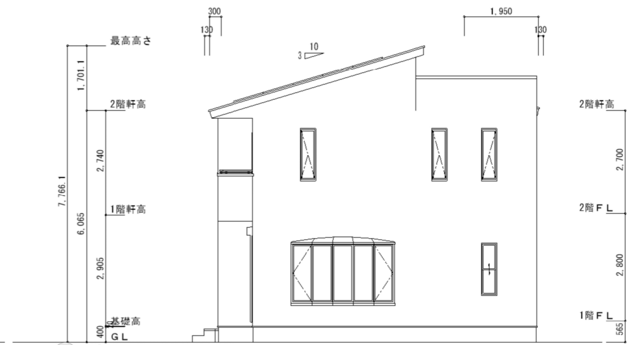
● 東面
